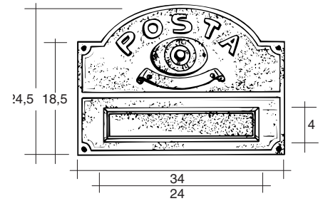
Dimensioni d'incasso - Recess dimensions
