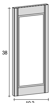
8083 Telaio porta moduli GALILEO da 3 moduli GALILEO module frame for 3 modules.
