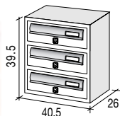
JUMBO 3 Blocchiera da 3 cassette 3 unit mailbox set
