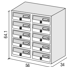
JUMBO 10 Blocchiera da 10 cassette 10 unit mailbox set
