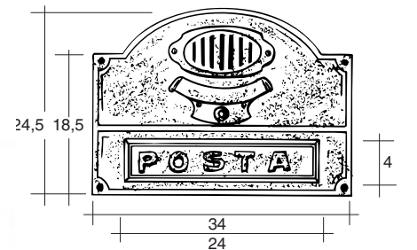
Dimensioni d'incasso Recess dimensions
