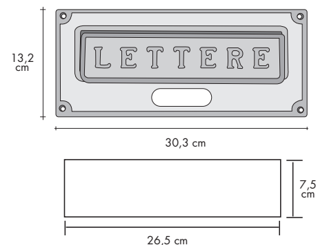
Dimensioni d'incasso - Recess dimensions
