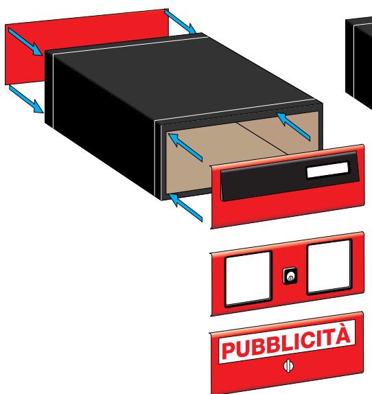
Composizione con mantello da recinzione Configuration with outer casing for fence mounting
