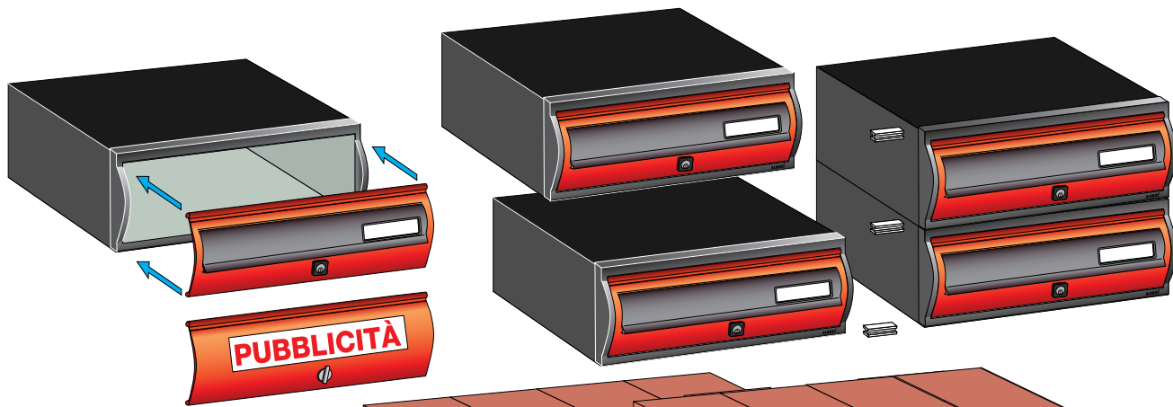
Composizione semincasso con mantello Configuration with outer casing for semi-recessed mounting
