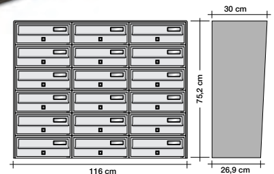
Esempio Slim con sportelli grigio antracite con elemento mobile ottone. Example of Slim with anthracite color doors and polished brass flap.
