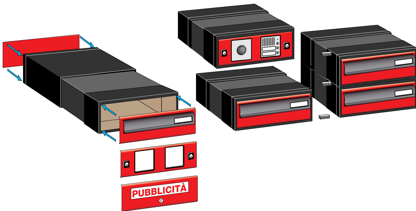
Composizione da incasso con doppia cornice coprifuga Configuration for recessed mounting with double external frame
