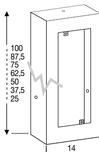
Placca porta accessori Intercom box
