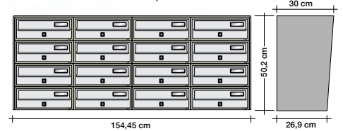
Esempio Slim con sportelli rossi. Example of Slim with red doors.
