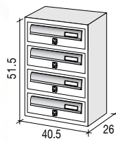
J4RO JUMBO 4 Blocchiera da 4 cassette 4 unit mailbox set
