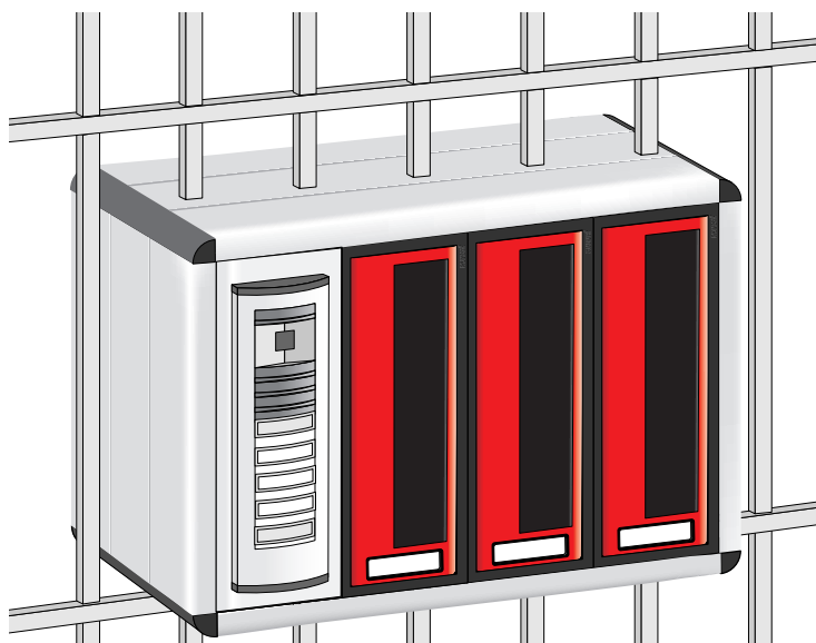
Composizione con mantello da recinzione Configuration with outer casing for fence mounting
