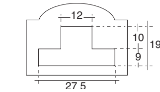
Dimensioni d'incasso - Recess dimensions
