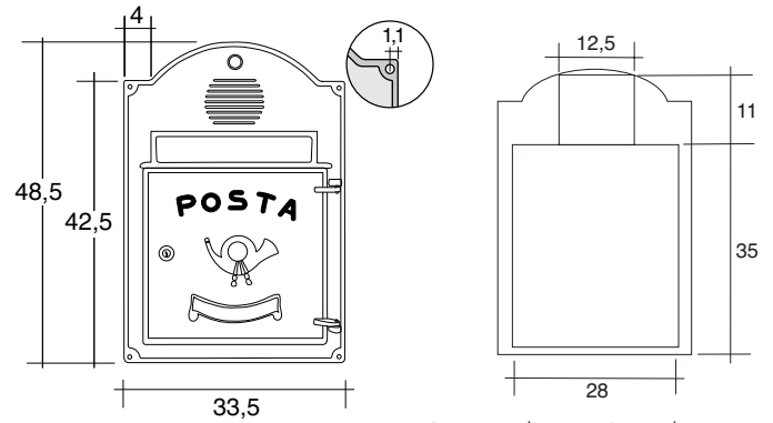
Dimensioni d'incasso - Recess dimensions
