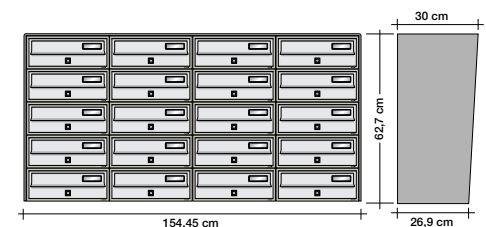
Esempio Slim con sportelli argento. Example of Slim with silver doors.
